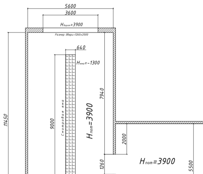
План помещения (гаражный бокс) ул. Северная д. 14
